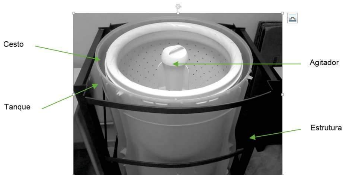
Representação esquemática do conjunto tanque-cesto-agitador
