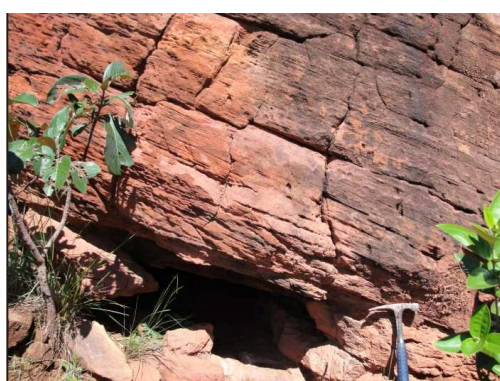
Estratificação cruzada em arenito
